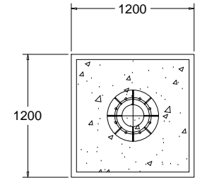
하부시공 상세도 SCALE: NONE
