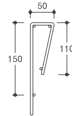
결곡 상세도 SCALE : NONE
