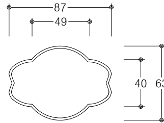
주주 상세도 SCALE : NONE
