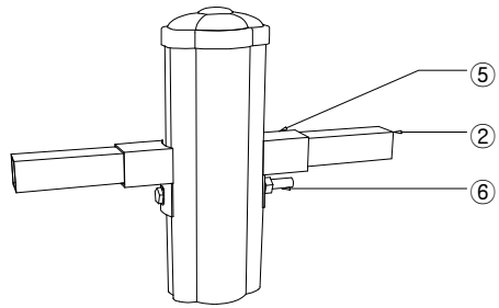
아트 조립도 SCALE : NONE
