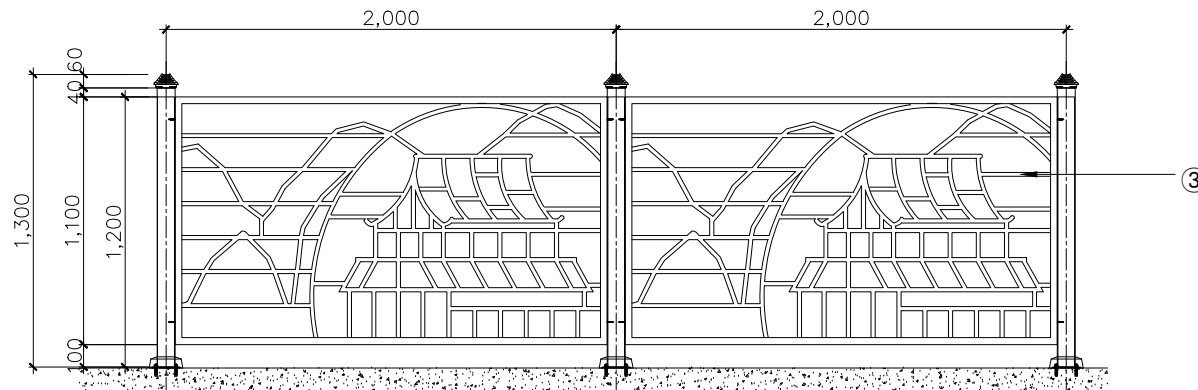
제품 상세도 SCALE : NONE
