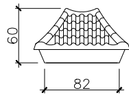
주주캡 정면도 SCALE : NONE
