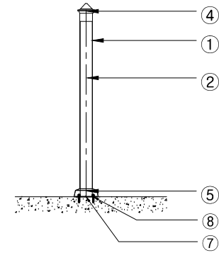
포스트 상세도 SCALE : NONE
